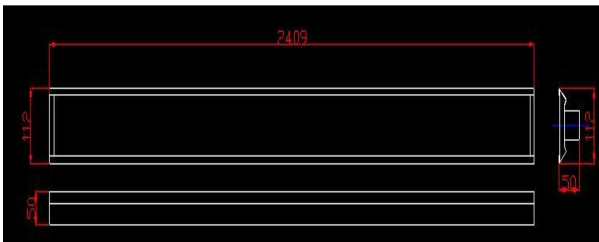
商店灯-8ft-80W/100W
