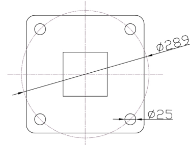
TEMPLATE (3:1)
